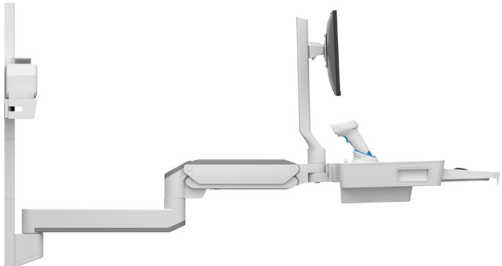
El sistema con superficie de trabajo y extensión opcional (98-547-251) alcanza los 165,7 cm
